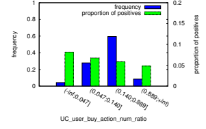
(d) user-category, rank 582
