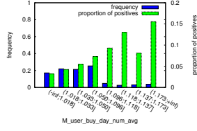
(d) merchant, rank 82
